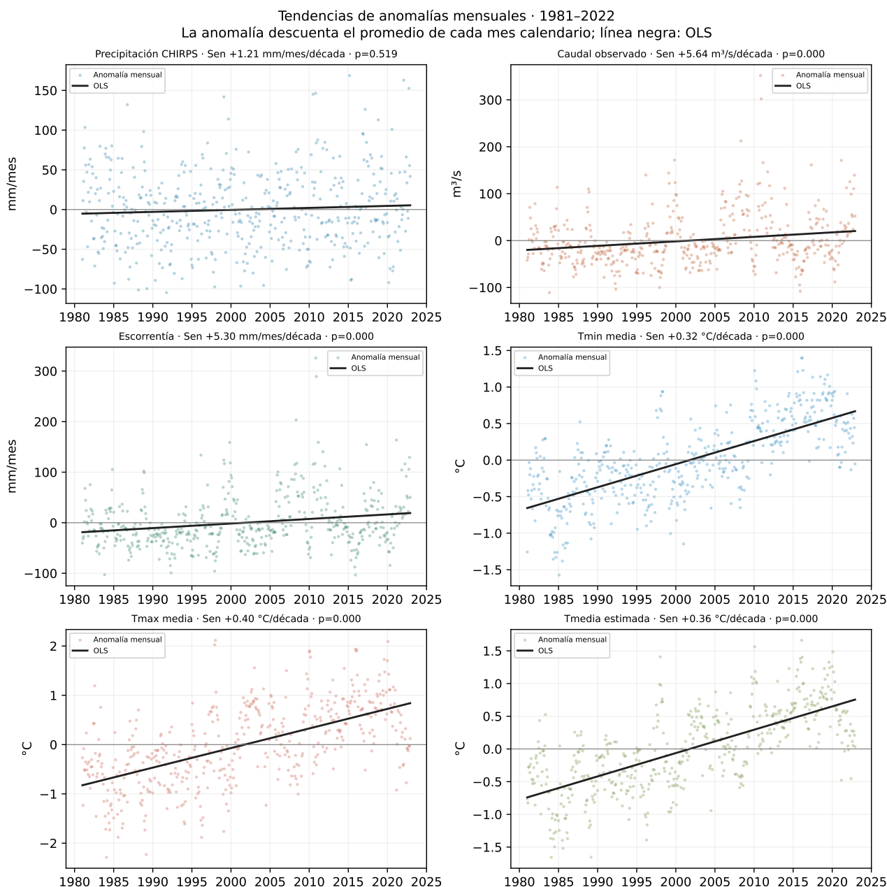
Figura 24: Anomalías mensuales y recta OLS, 1981–2022. Los títulos presentan la pendiente de Sen estacional por década y el valor p de Mann–Kendall estacional.
